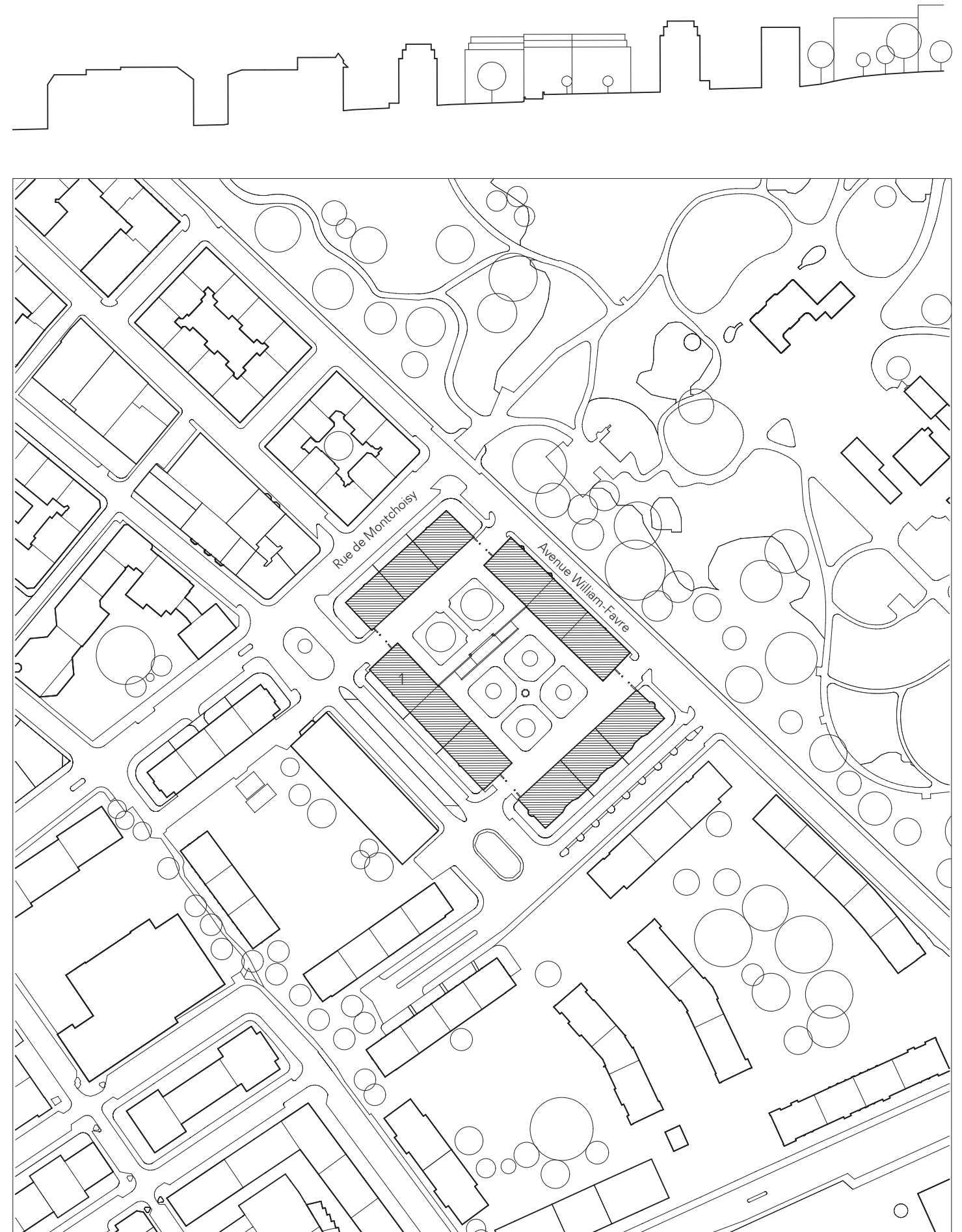
Square Montchoisy Plan masse — 1:2000
